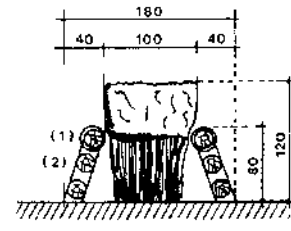
Double barrière
